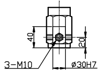
S 部詳細
